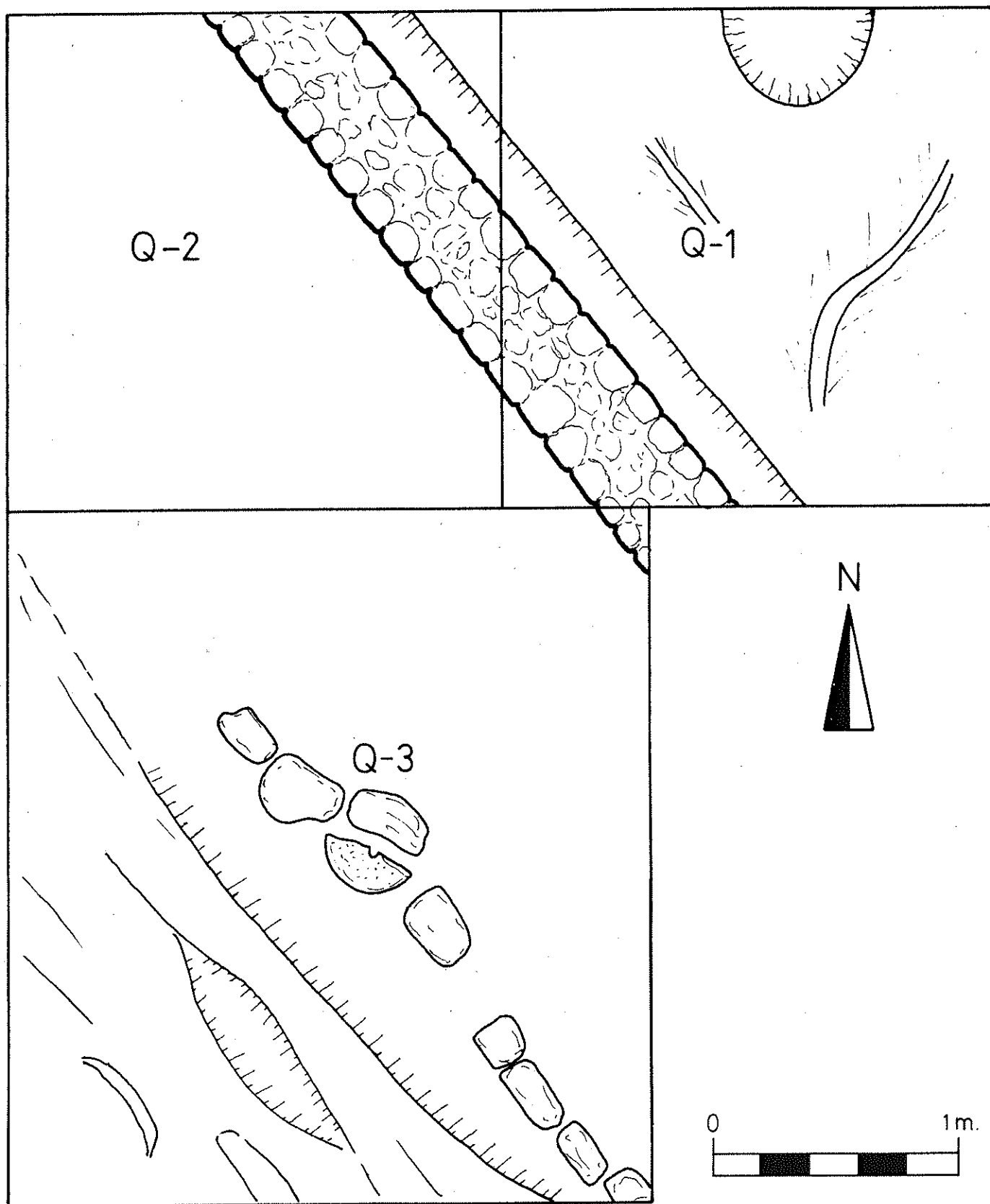
LAM. 4 Planta del templeig
