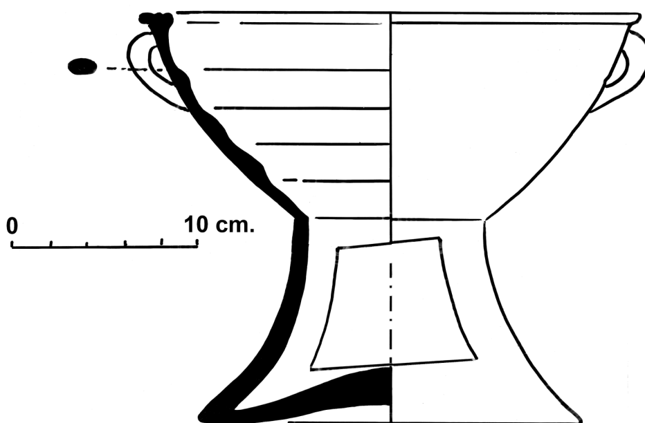
Dibuix en secció del fogó de ceràmica.
