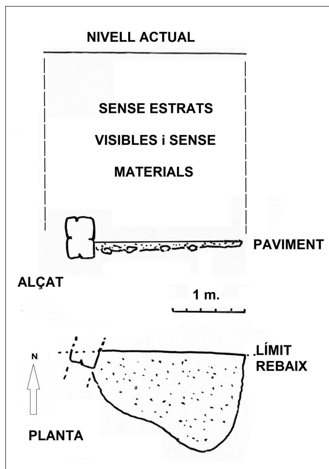
Figura 8: La Riera, 7 - 13, alçat i planta de les restes.
