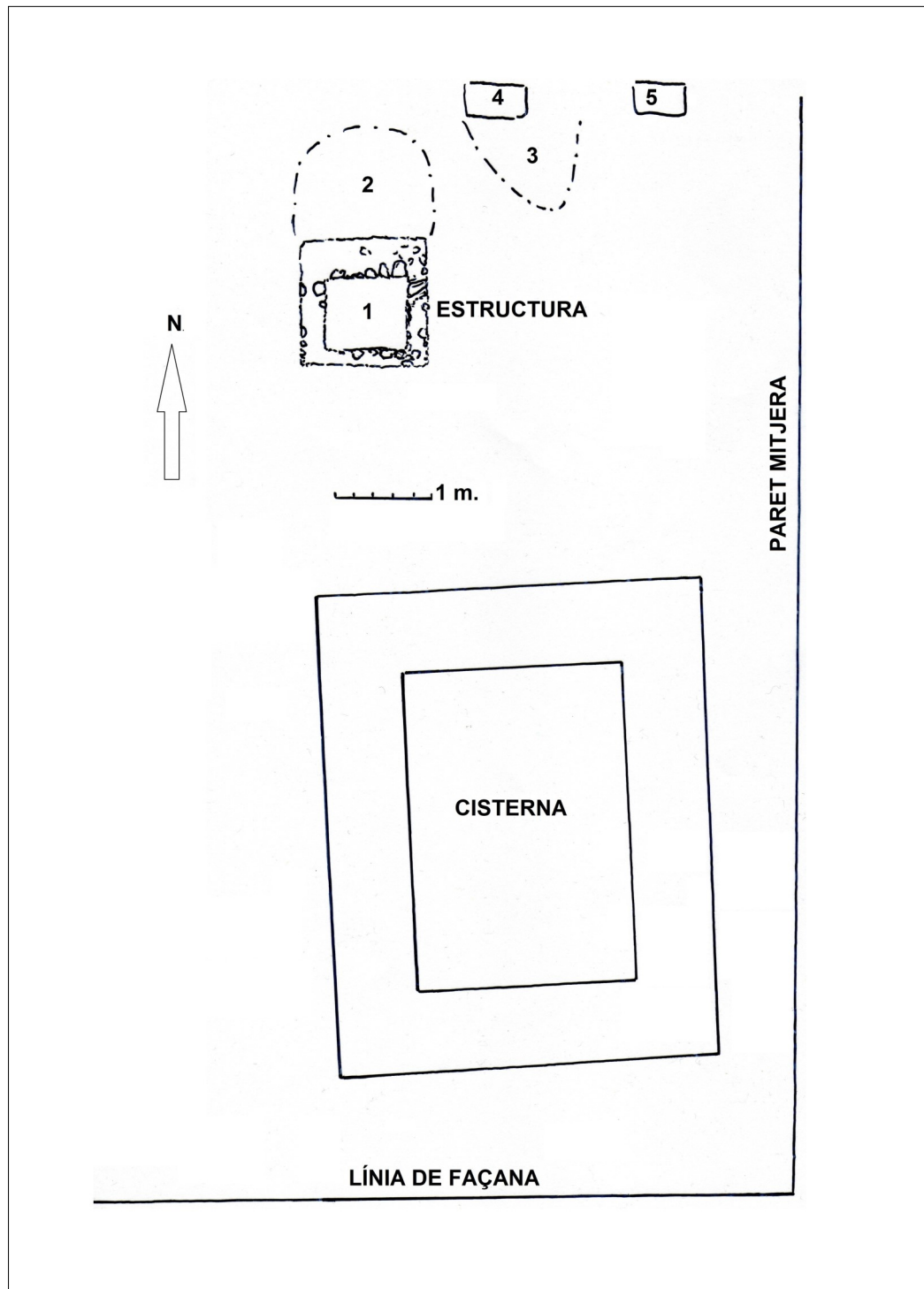
Figura 1: c/ Nou, 27, planta de les restes.
