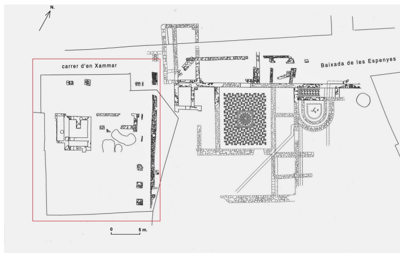
Figura 2: Planta de les termes de can Xammar i la palaestra de can Damia (dibuix: Cela-Garcia-Pera 2003).
